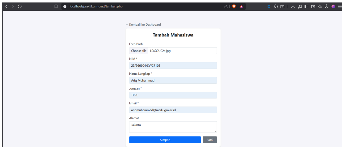
Gambar 6. Tampilan tambah.php
